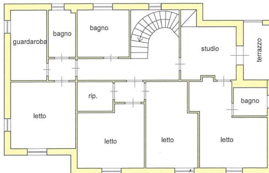
PIANO PRIMO H: 2.70
