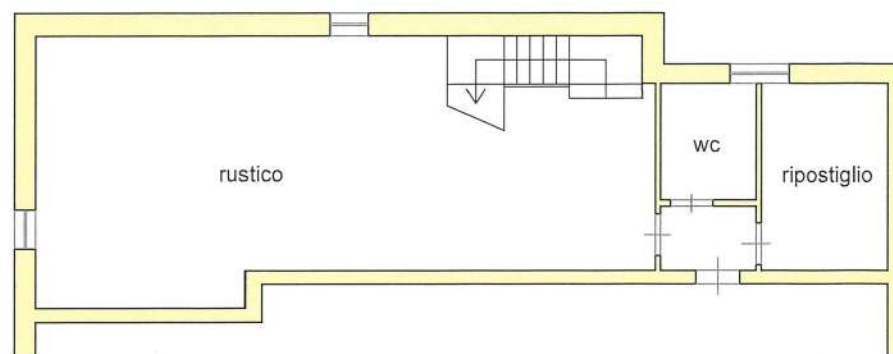
PIANO PRIMO SOTTOSTRADA H: 2.50
